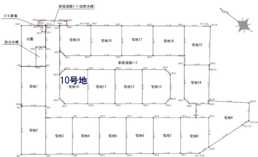
【区画図】
