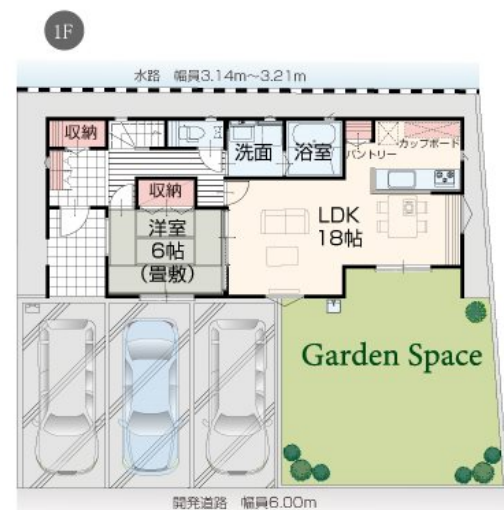
【間取り図】
