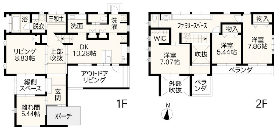
【間取り図】
