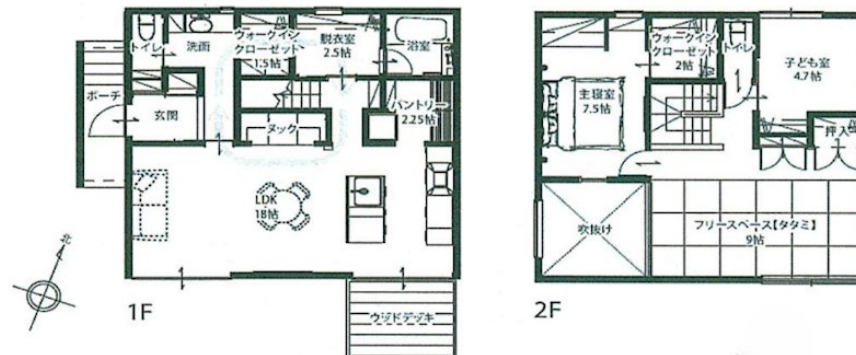
【平面図】
