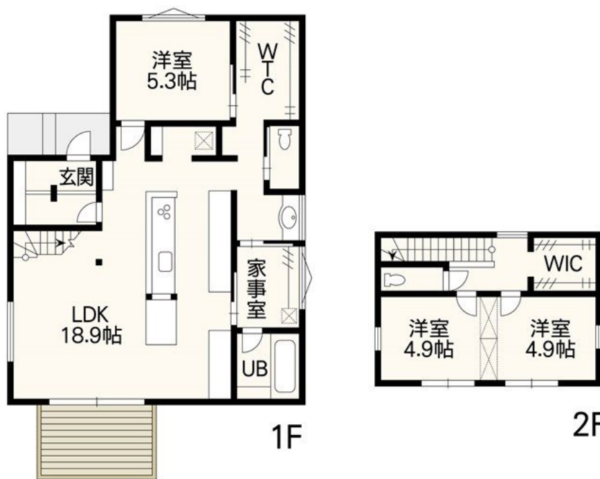
【間取り図】
