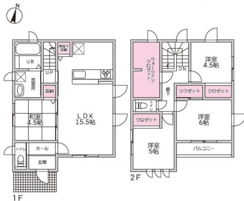
【間取り図】
